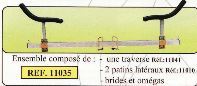
Ensemble support patin de nez réglable avec caoutchouc et brides
