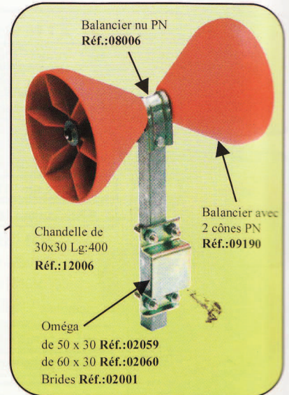
Ensemble cônes sur balancier avec chandelle, brides et oméga
