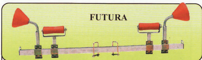
Ensemble composé de : - une traverse Réf.:11041 - 2 ensembles Réf.:11070 - brides et omégas
